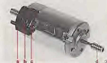
Bild 3 LGB-Hochleistungsmotor a) Herausgezogener Isolierkopf mit Führungskanal für Motorkohlen b) Drossel-Spulen zur Funkentstörung c) Zweigängige Getriebeschnecke. Motor-Leistungsdaten (Durchschnittswerte) Drehmoment M_d = 0,4-0,6 \text{ Ncm}^* Drehzahl n = 7000-11000 \text{ U/min} Stromaufnahme J = 300-500 \text{ mA} Leistung P_{ab} = 3-7 \text{ Watt} Motor-Wirkungsgrad \eta = 67\% Alle Meßwerte bei mittlerer Zugleistung mit 10 Wagen in der Ebene. * (1 Newton ca. 100 g)
